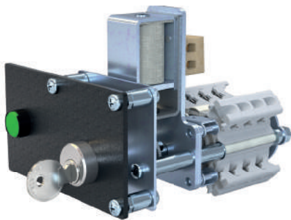
SR105 Solenoid lock switch SR105 con interblocco elettromeccanico
